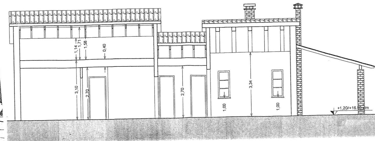
SEZIONE X-X
