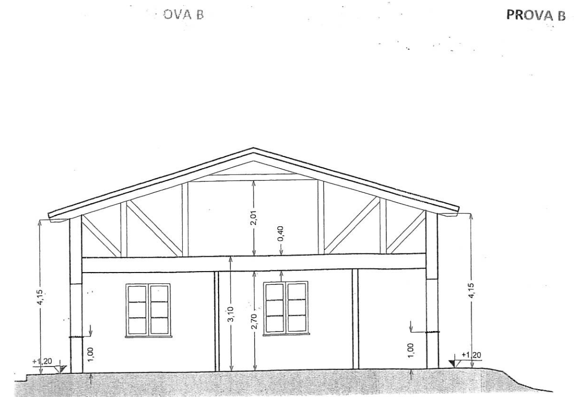
SEZIONE W-W
